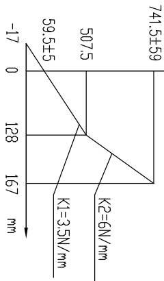
弹簧特性图
